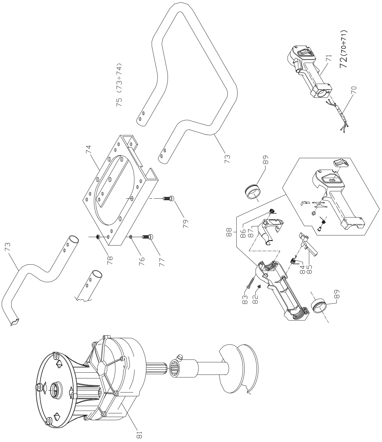
Fig. 6 (T- 160HO)
